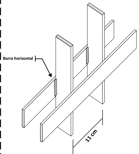
DETALHE A Montagem Dupla das Barras
